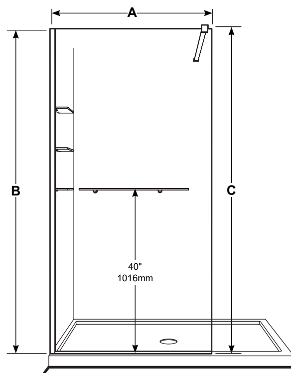
front view / Vue de face
