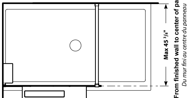
Top view / Vue de dessus
