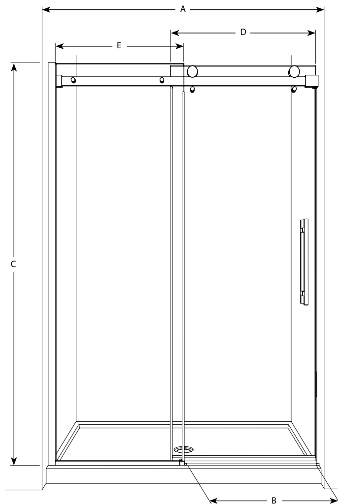
Front view / Vue de face
