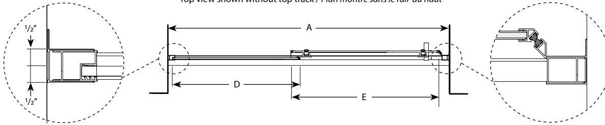
Top view shown without top track / Plan montré sans le rail du haut
